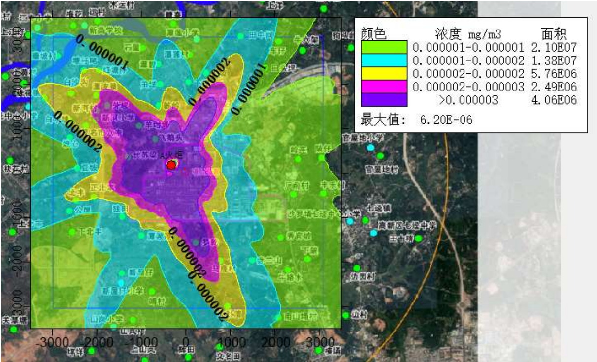
图 5.1-13 PM 10 日均最大落地浓度贡献值分布图
