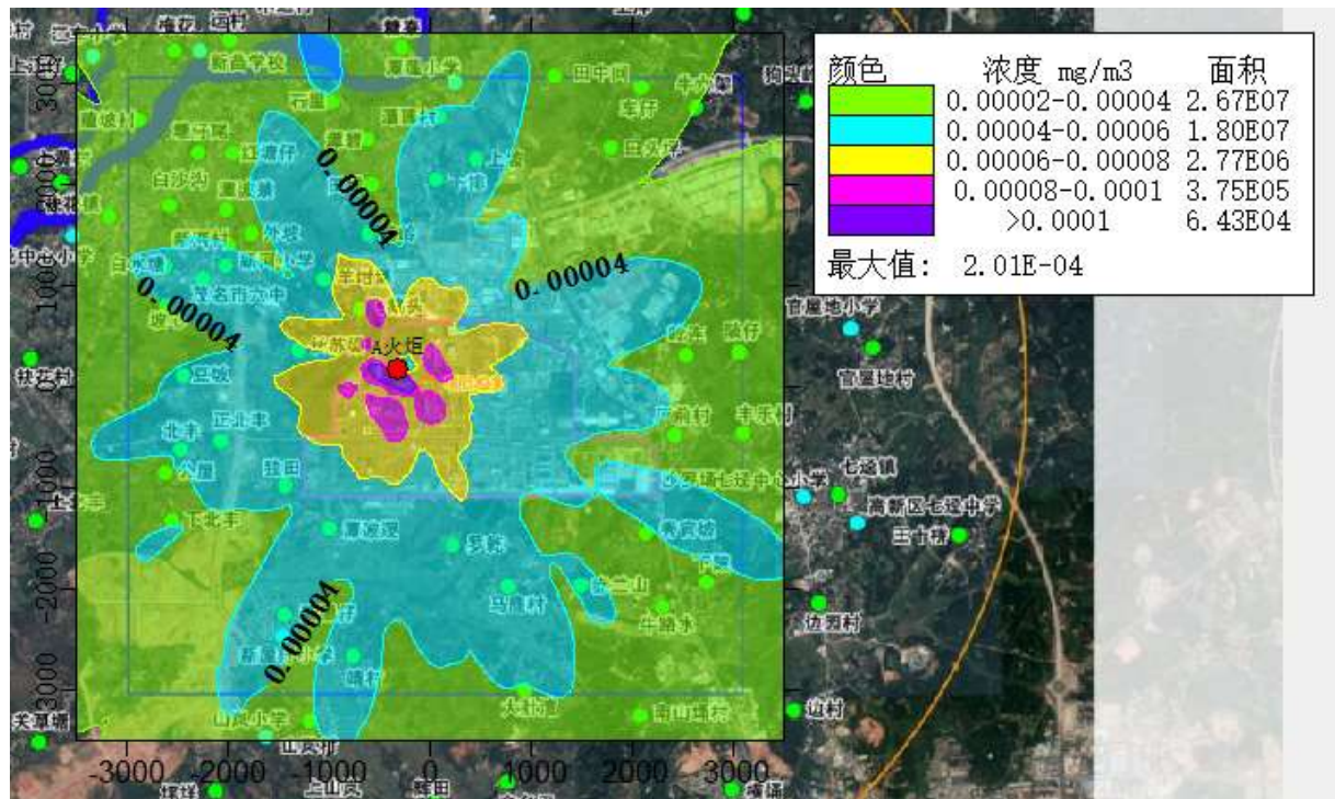
图 5.1-10 NO 2 小时最大落地浓度贡献值分布图
