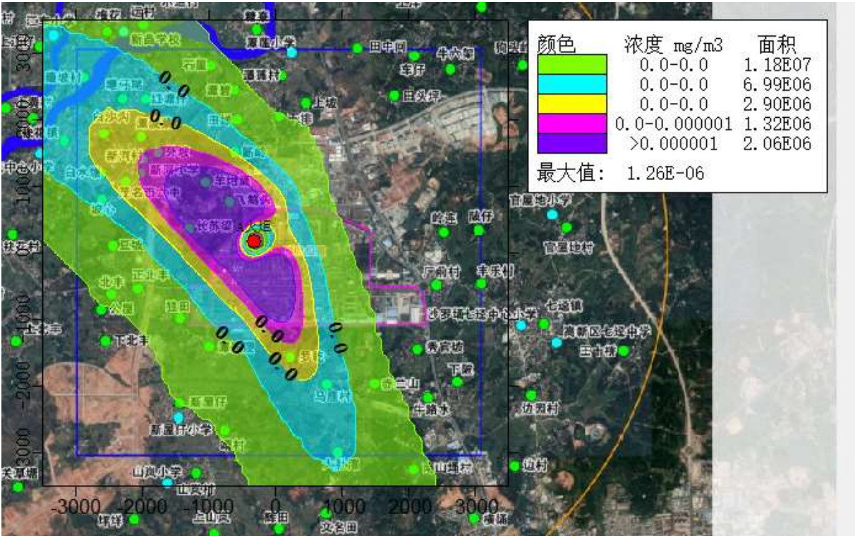
图 5.1-14 PM 10 年均最大落地浓度贡献值分布图
