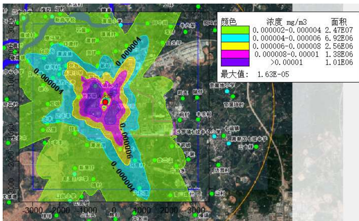
图 5.1-11 NO 2 日均最大落地浓度贡献值分布图
