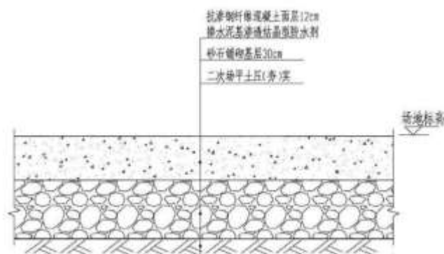
图 6.5-1 一般污染防治区防渗结构示意图
