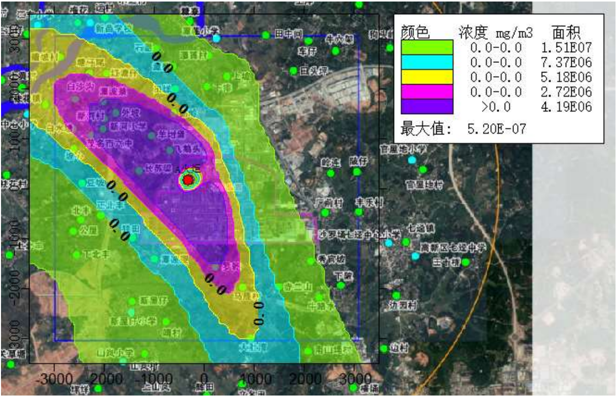
图 5.1-9 SO 2 年均最大落地浓度贡献值分布图
