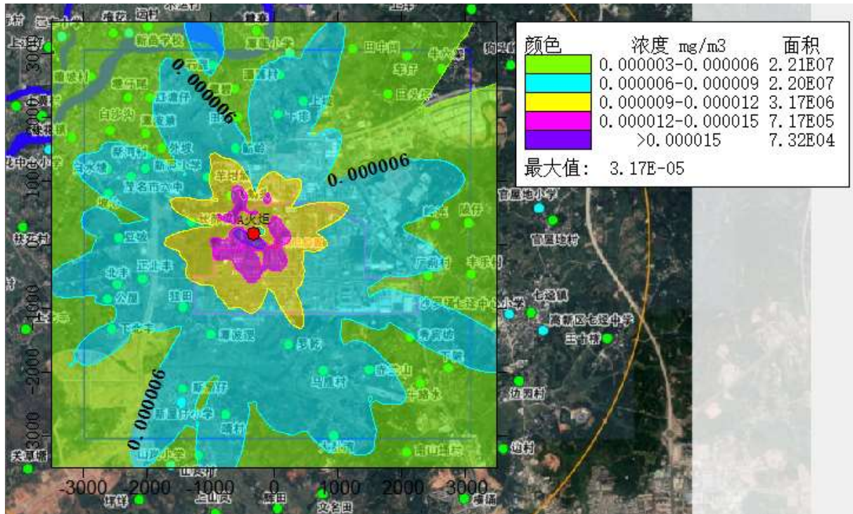
图 5.1-7 SO 2 小时最大落地浓度贡献值分布图
