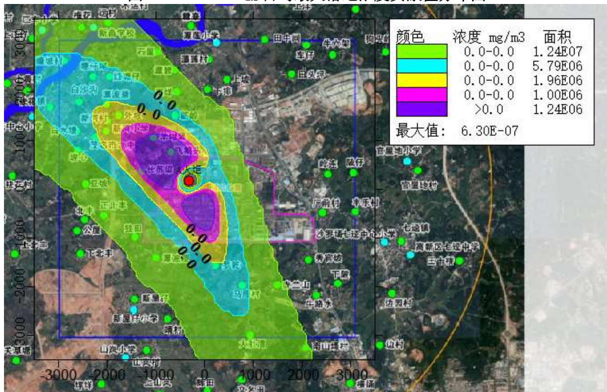
图 5.1-16 PM 2.5 年均最大落地浓度贡献值分布图
