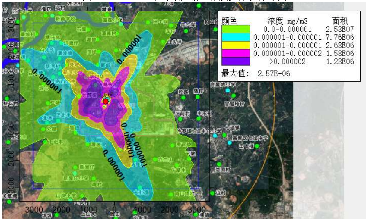
图 5.1-8 SO 2 日均最大落地浓度贡献值分布图
