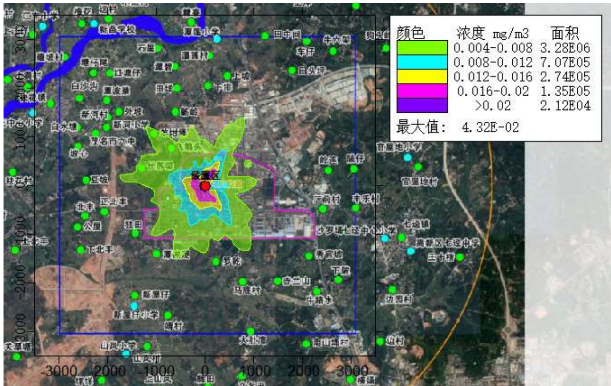
图 5.1-17 VOCs8 小时平均最大落地浓度贡献值分布图
