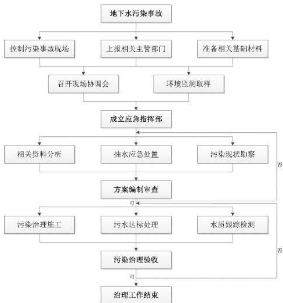
图 6.5-2 地下水污染应急治理程序
