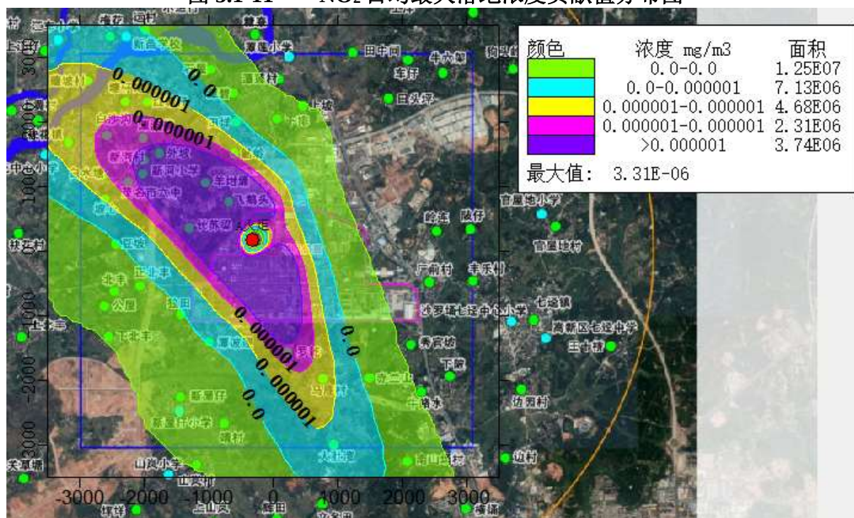
图 5.1-12 NO 2 年均最大落地浓度贡献值分布图
