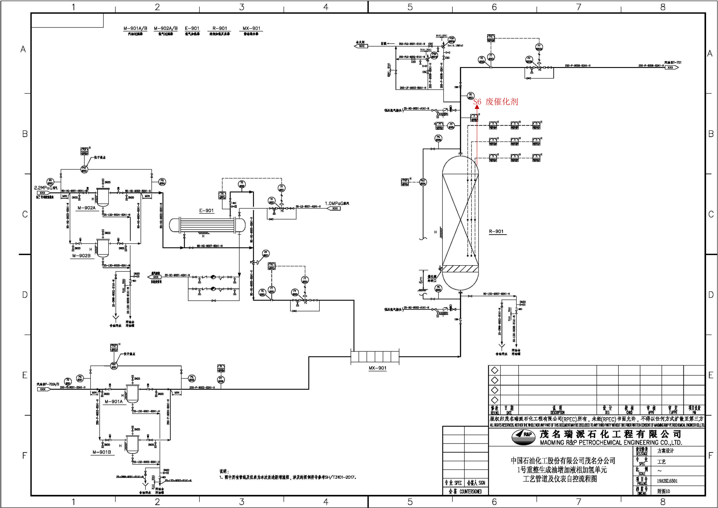
图 3.2-3b 1#重整装置新增液相加氢单元工艺流程及产污环节图
