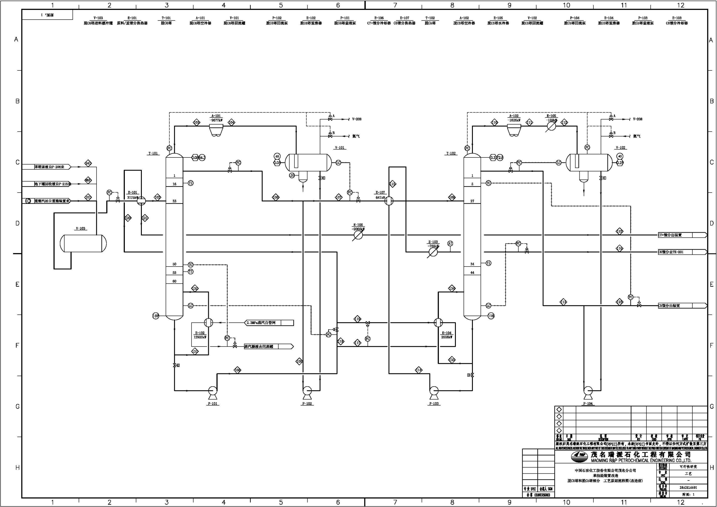
图 3.2-2b 苯抽提装置脱 C6 塔和脱 C5 塔工艺流程及产污环节图（改造前）
