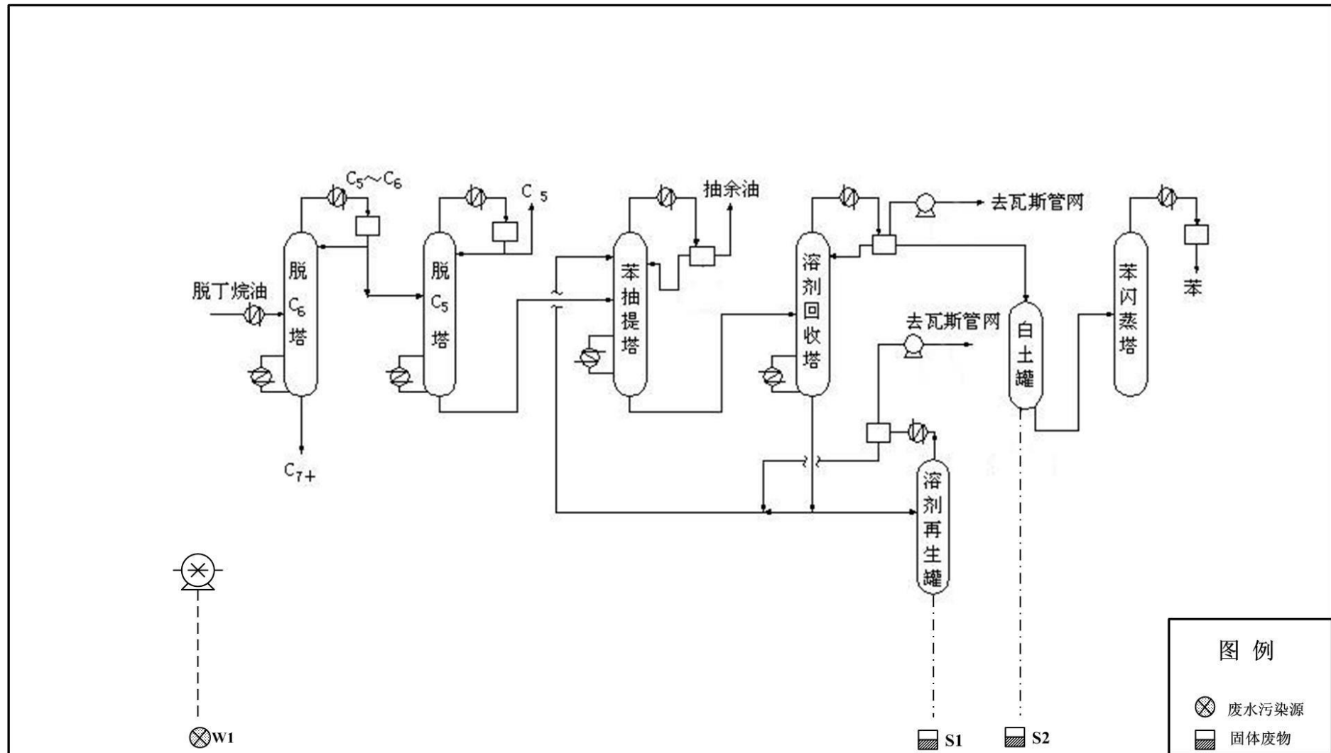
图 2.2-1 现有苯抽提装置工艺流程图
