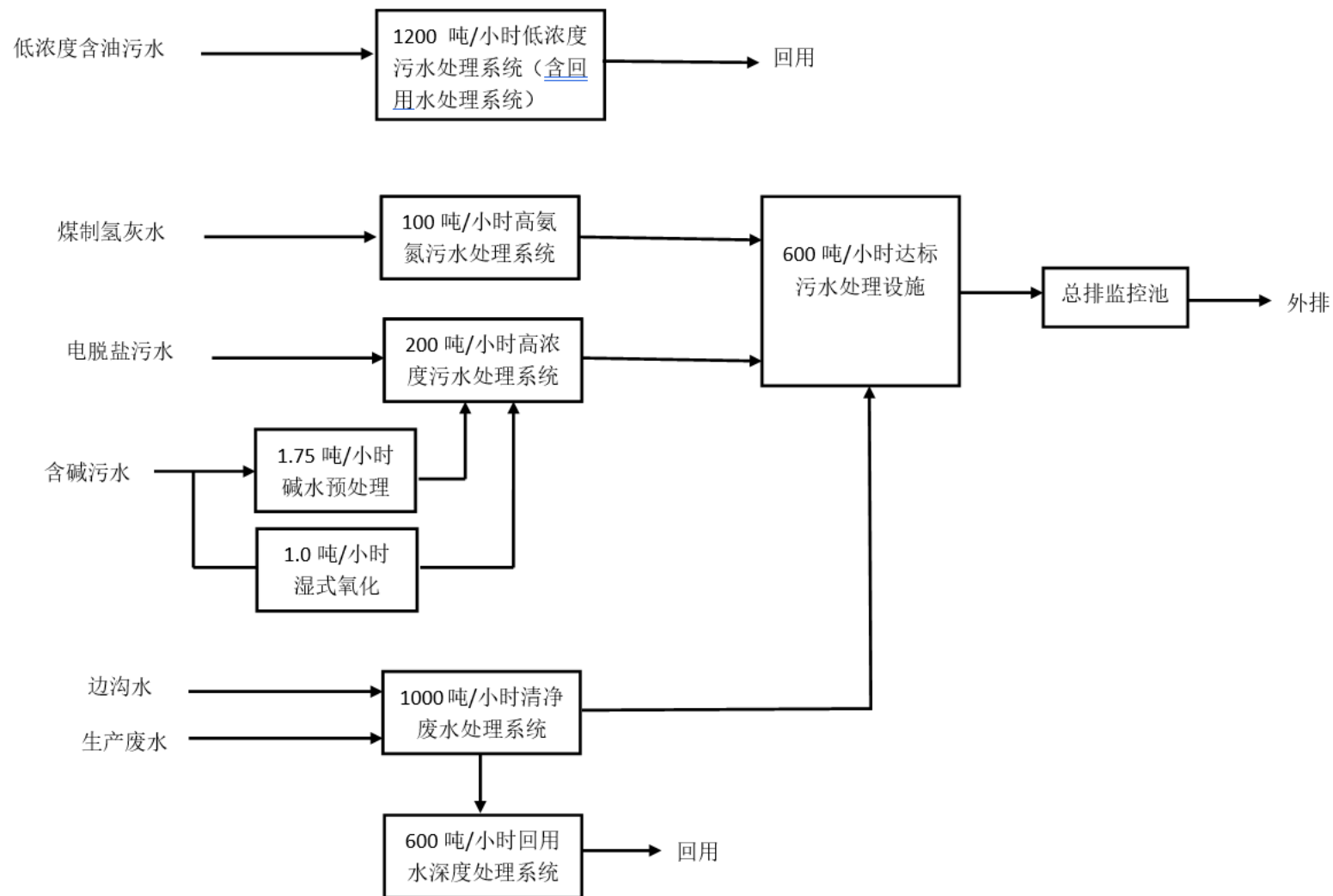
图 6.2-1 炼油厂区污水处理场系统的走向示意图
