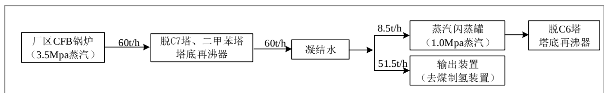
图 3.3-2 蒸汽平衡情况
