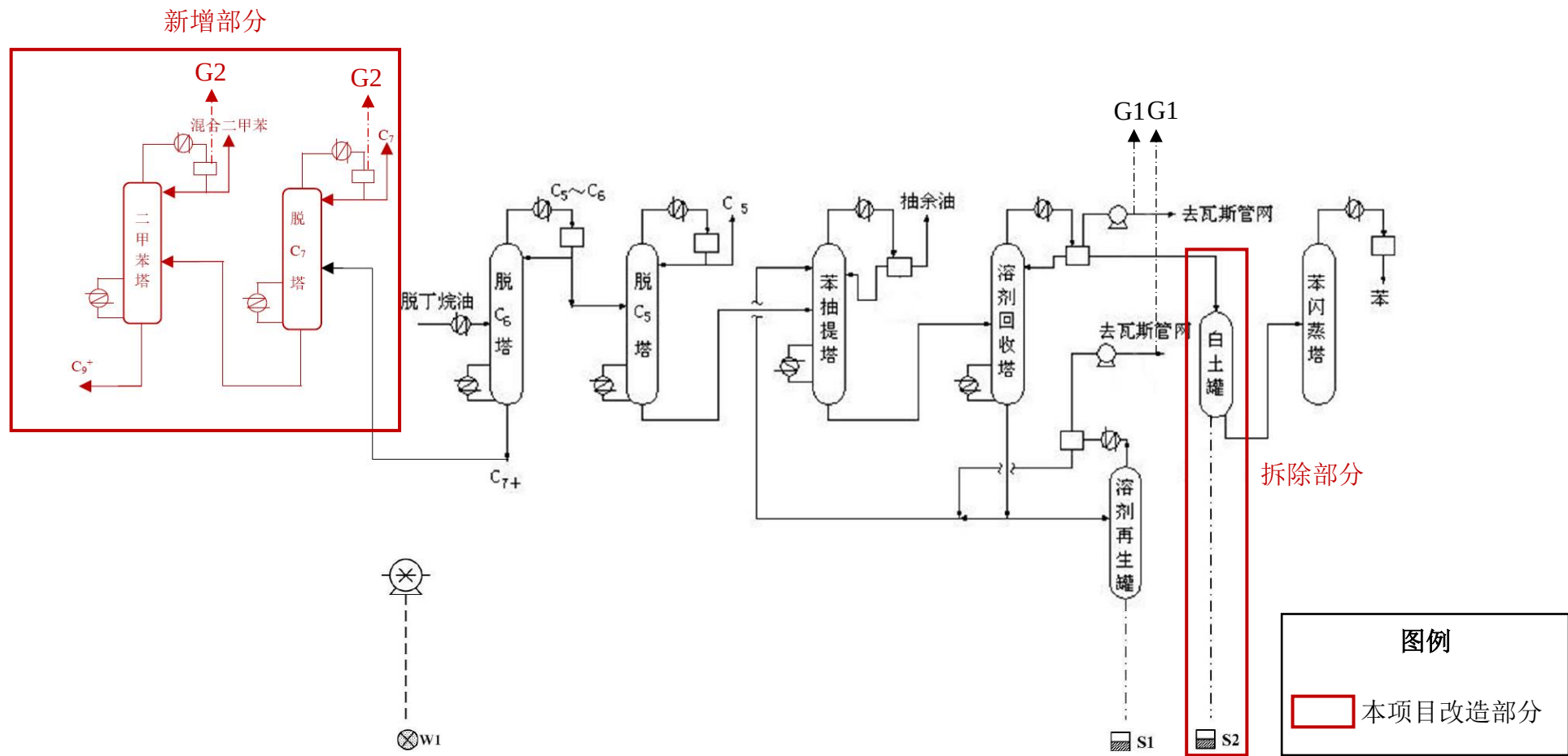
图 3.2-2a 苯抽提装置工艺流程及产污节点图（改造后）
