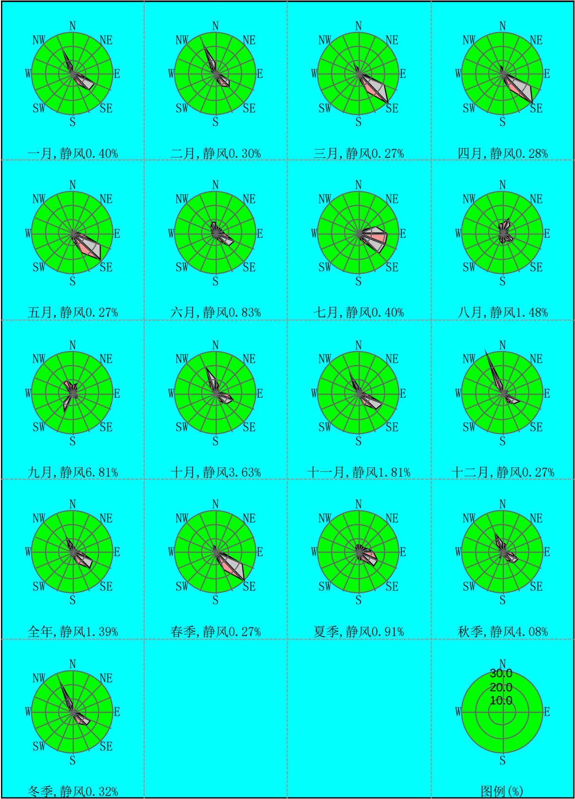
图 5.1-5 2018 年项目所在区风玫瑰图
