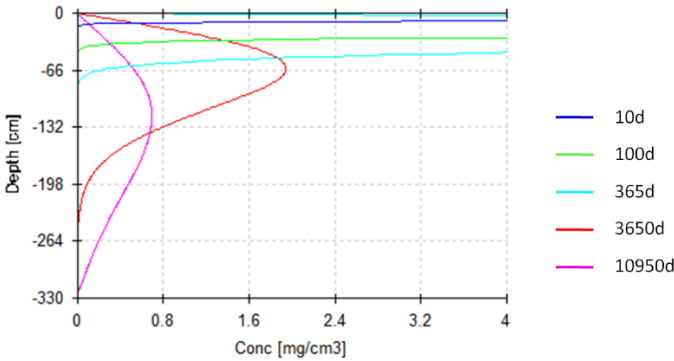
图5.7-1 包气带中二甲苯污染质运移浓度深度变化图
