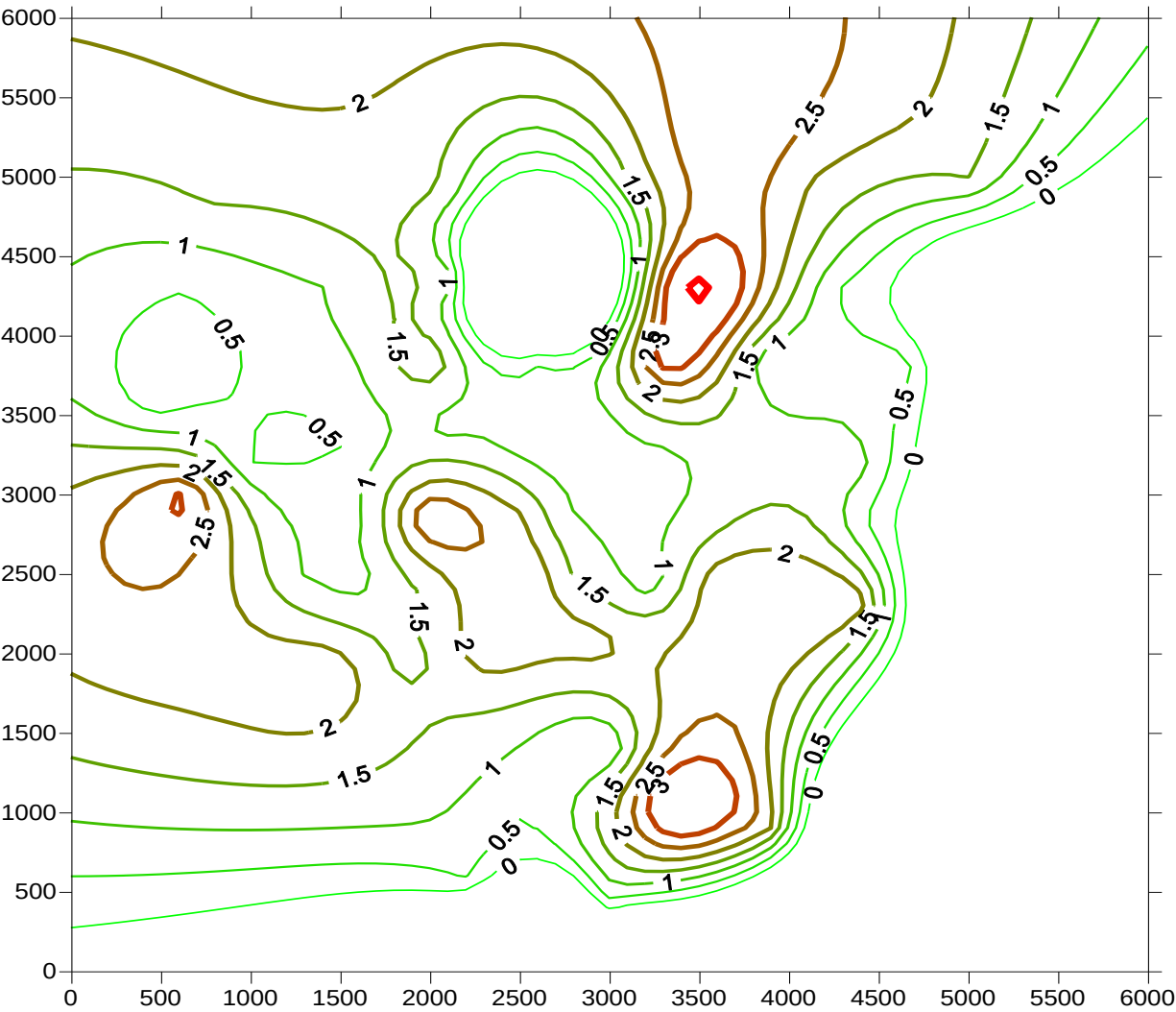
图 5.3-1 包气带厚度等值线图
