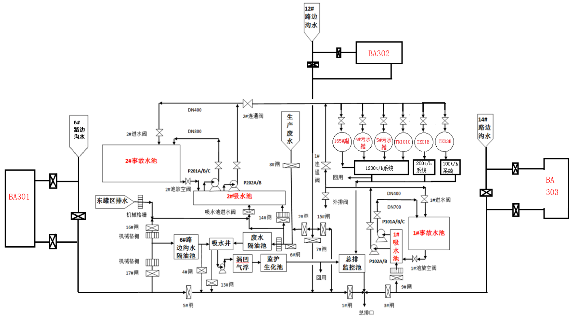
图 5.6-3 茂石化炼油厂三级事故水收集处理示意图
