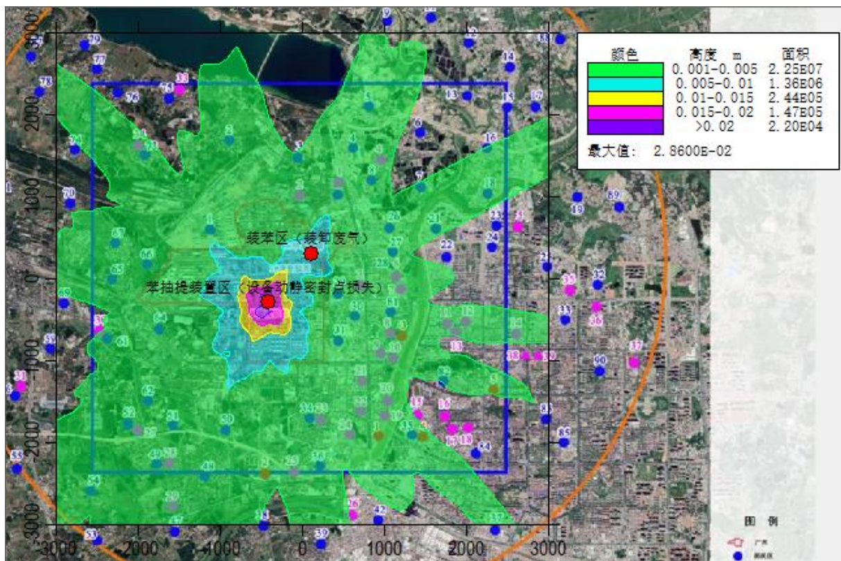
图 5.1-8 VOCs 日均最大落地浓度贡献值分布图
