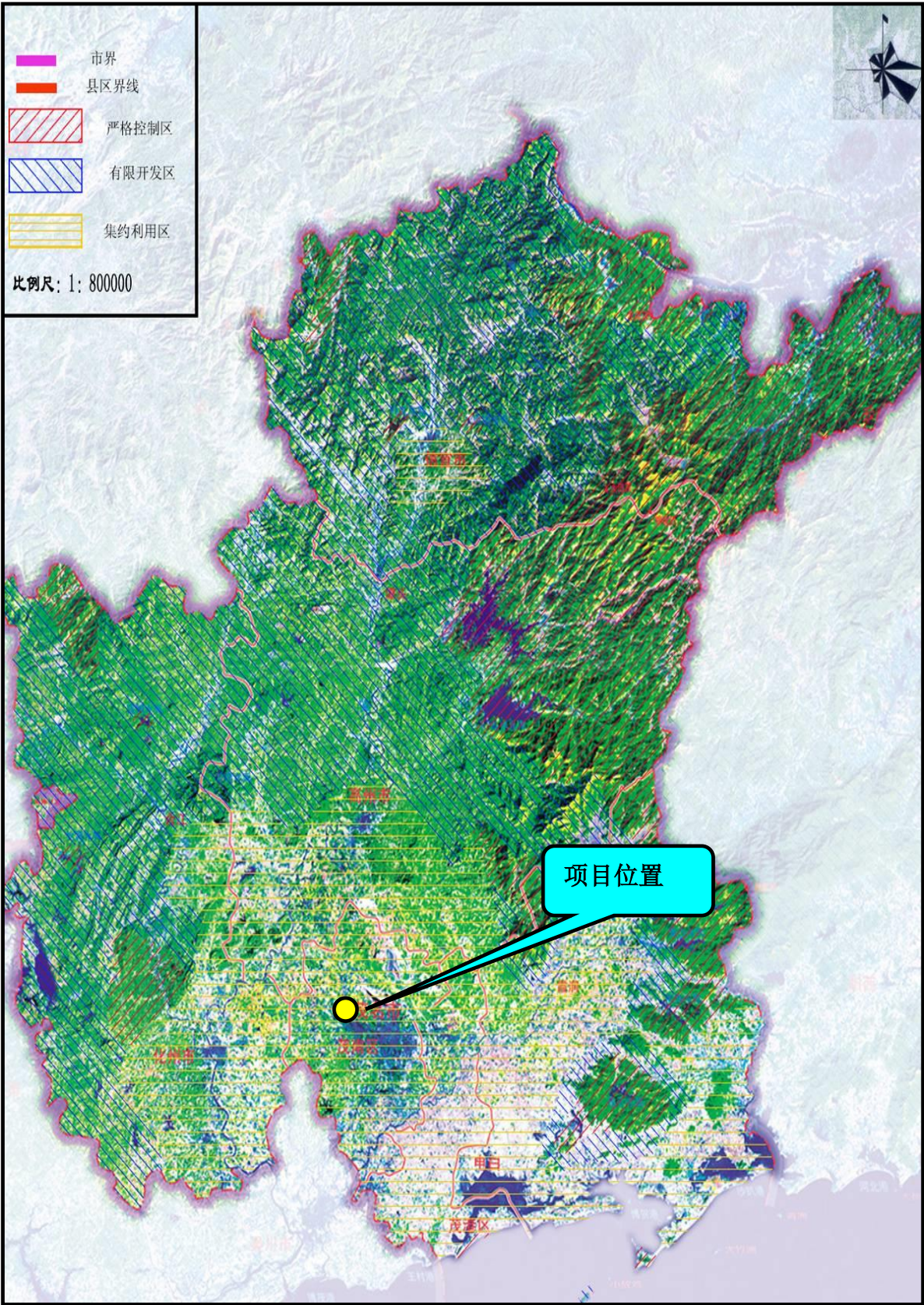
图 1.2-4 茂名市生态分级控制规划图
